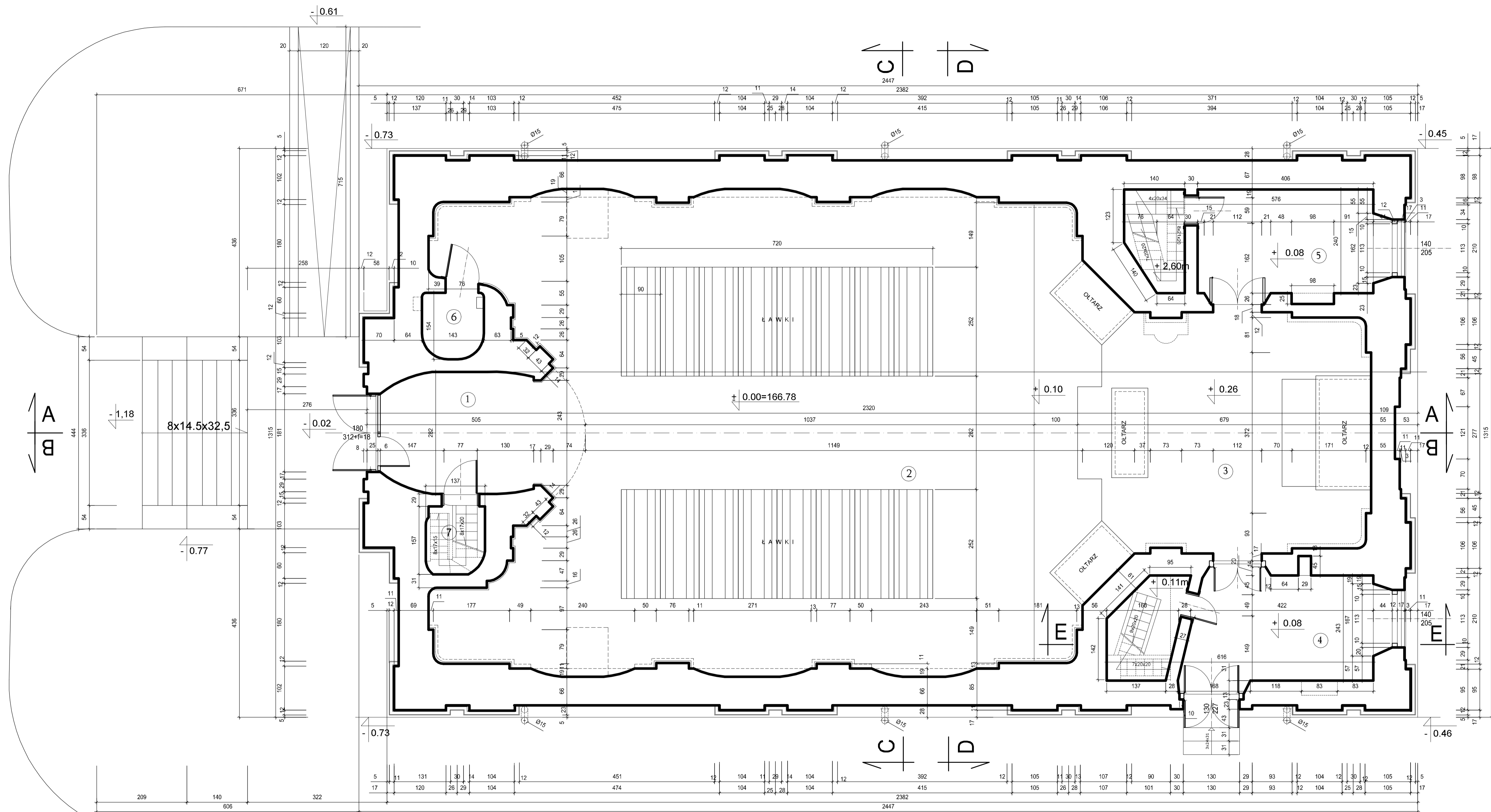
RZUT PRZYZIEMIA - POZIOM 0 SKALA 1:50
