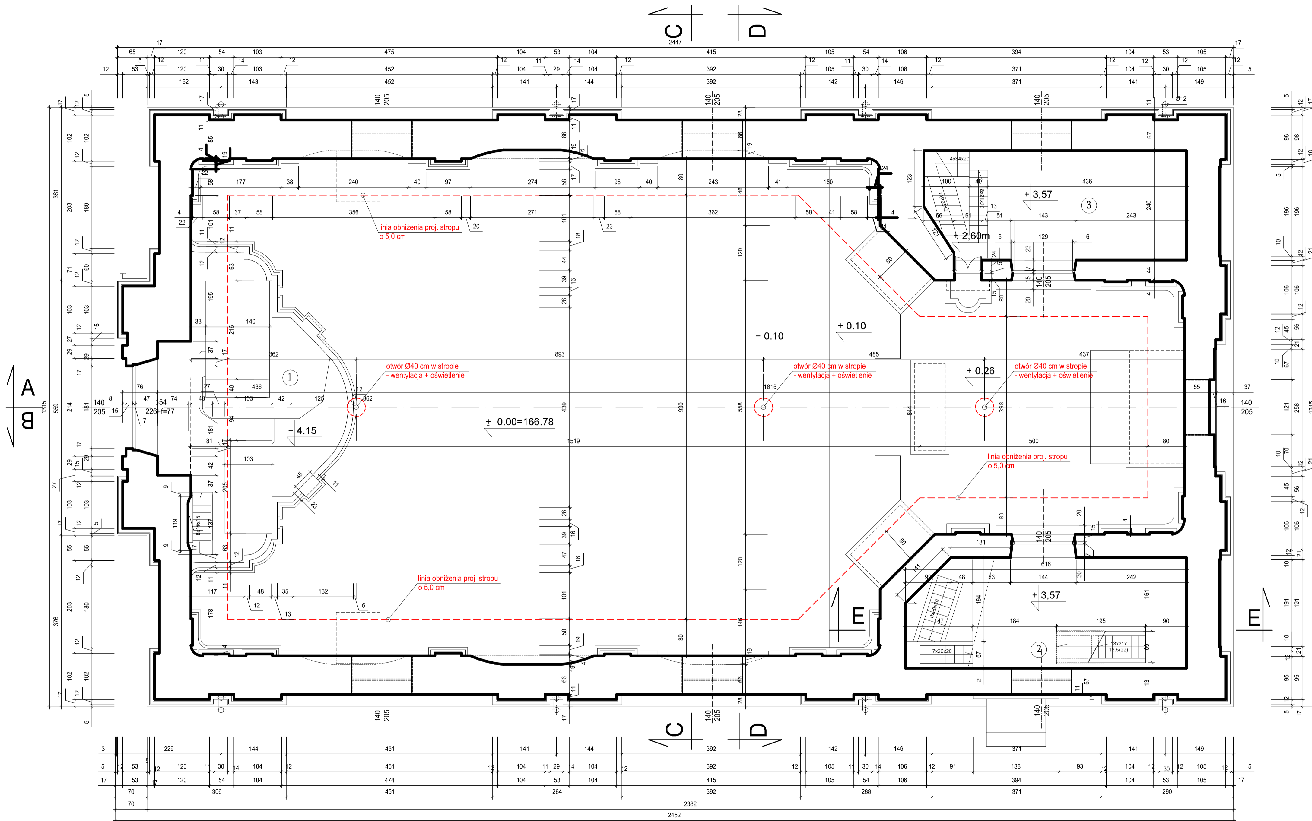
RZUT CHÓRU - POZIOM I SKALA 1:50
