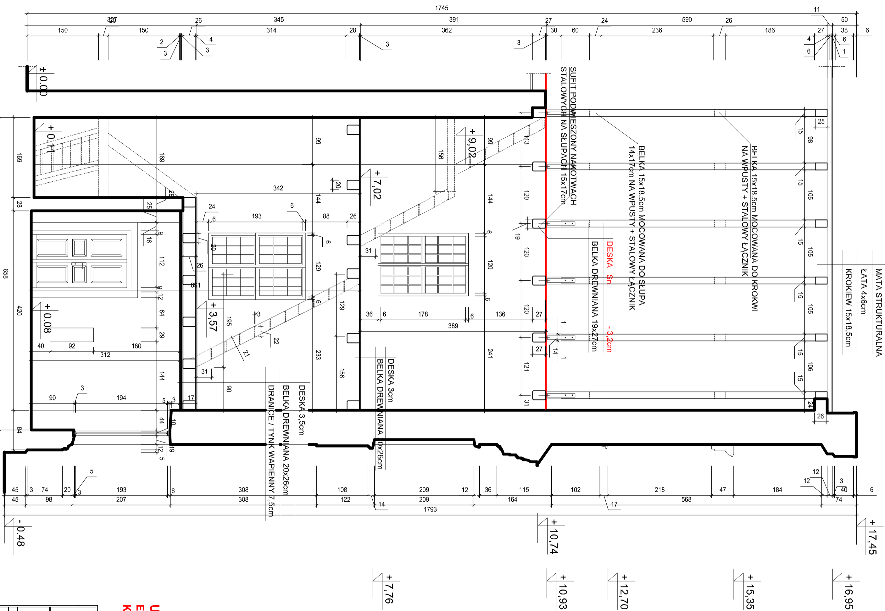
PRZEKRÓJ E - E SKALA 1:50
